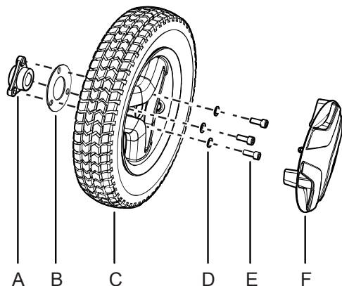
Abbildung 192. Montieren des Antriebsrads.
