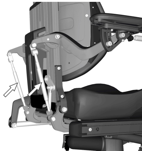
Abbildung 131. Armlehnenwinkel, Einstellungsleisten.
