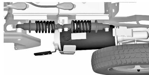
Abbildung 20. Antriebseinheit und Stoßdämpfer.
