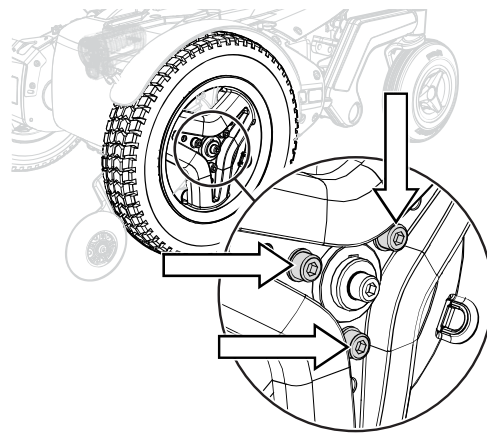
Abbildung 199. Verwenden Sie einen Drehmomentschlüssel zum Anziehen der Schrauben.
