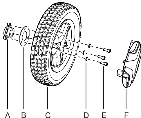
Abbildung 191. Montieren des Antriebsrads.
