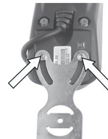
Abbildung 141. Entfernen Sie nur eine der Schrauben.
